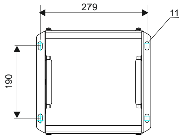
Befestigungslochbild Ansicht von unten
